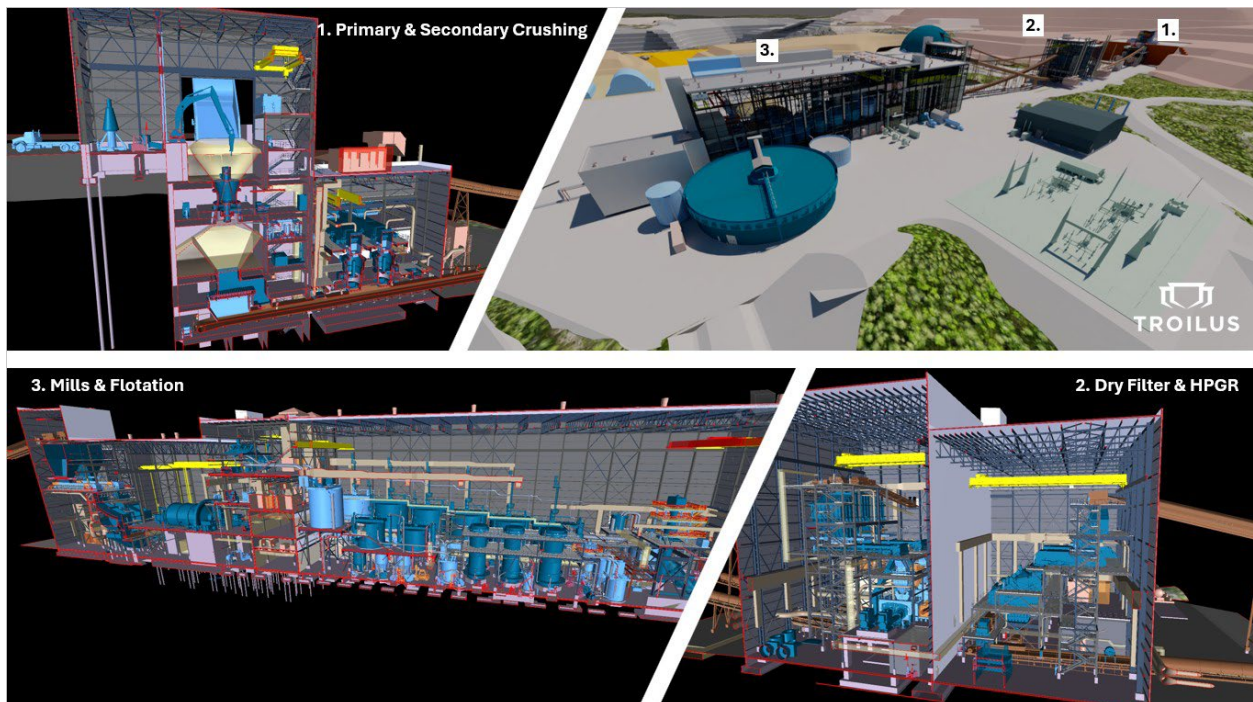
Figure 1. Projet Troilus – Modèle 3D du circuit de traitement
